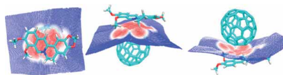
Рис. 2. Расчетные электронные плотности при возможном комплексообразовании фуллерена C 70 и противоопухолевого препарата на основе берберина.
